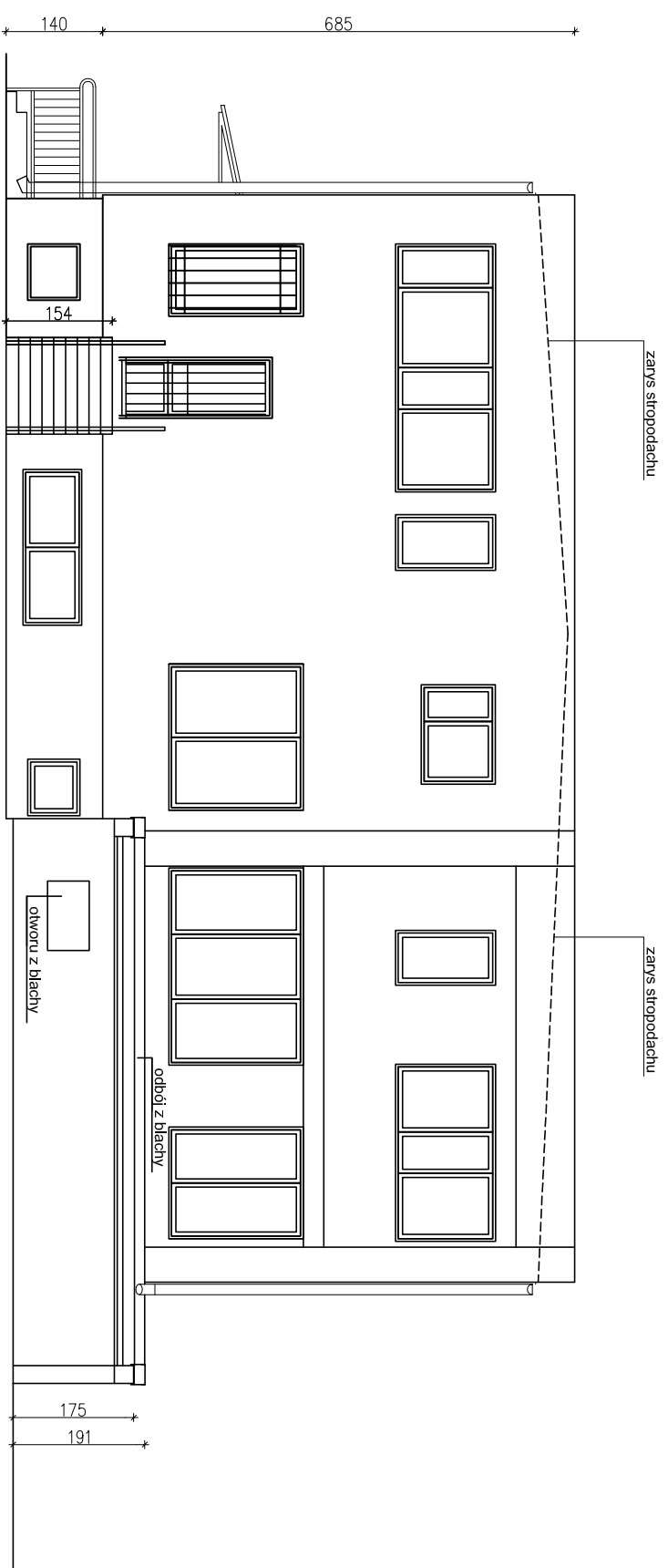
ELEWACJA ZACHODNIA 1:100
